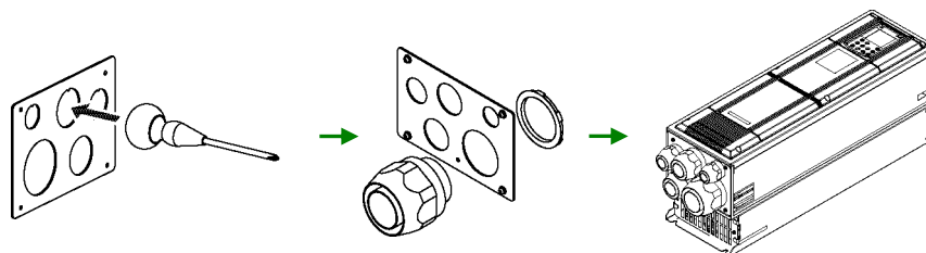
Abb. 2.3 Ausstanzen von Löchern im Klemmenblock und Anbringung von Kabelverschraubungen bzw. Leitungen.
