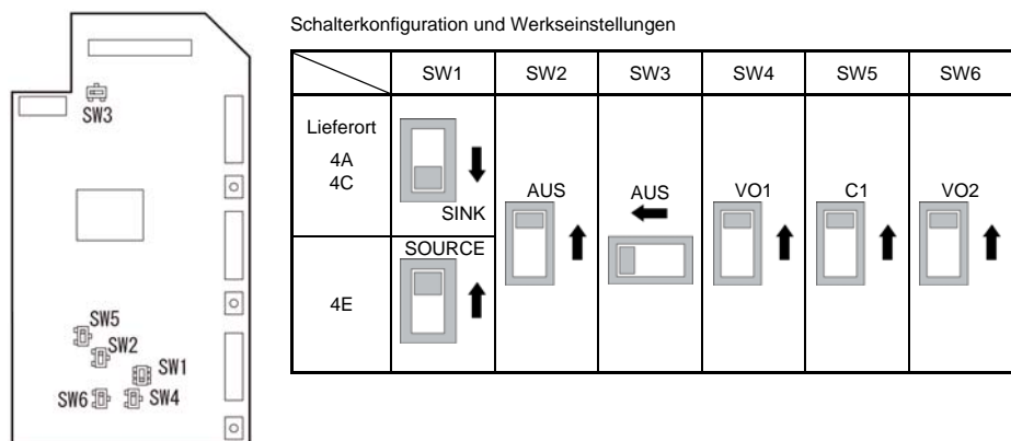
Abbildung 2.4 Anordnung der Schiebeschalter auf der Steuerungsplatine
